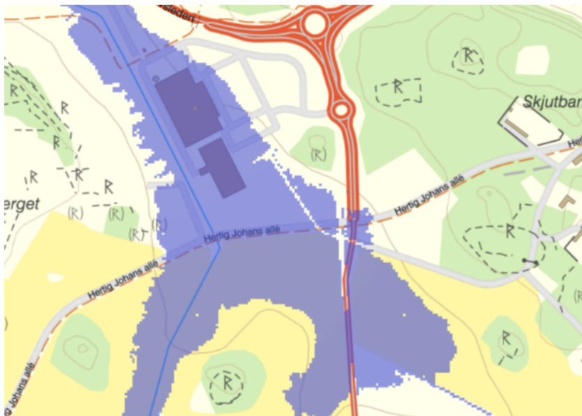
Figur 9. Översvämning av Djurgårdens centrum vid beräknat högsta flöde i Tinnerbäcken.
