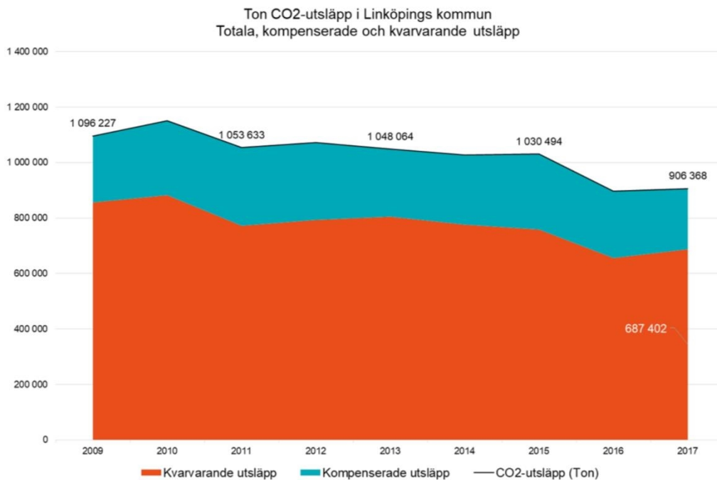
Figur 3. Ton koldioxidutsläpp i Linköpings kommun. Totala, kompenserande och kvarvarande utsläpp. Årligen 2009-2017.
